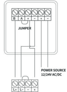
3. CONNEXIÓ DE BLOQUEIG ESTÀNDAR MOTORIZAT
