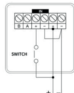
3. SENYAL AMB TANCAMENT A MASS
