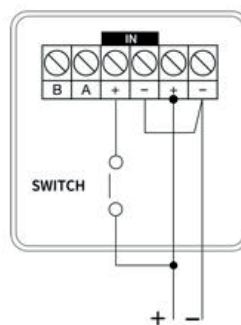
2. SENYAL AMB TANCAMENT EN FONT D'ALIMENTACIÓ
