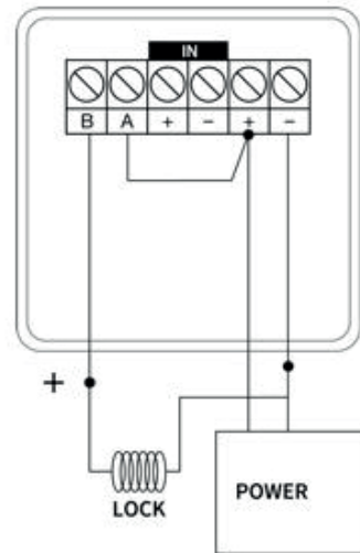
2. CONNEXIÓ DE BLOQUEIG ELECTROMEQUIC
